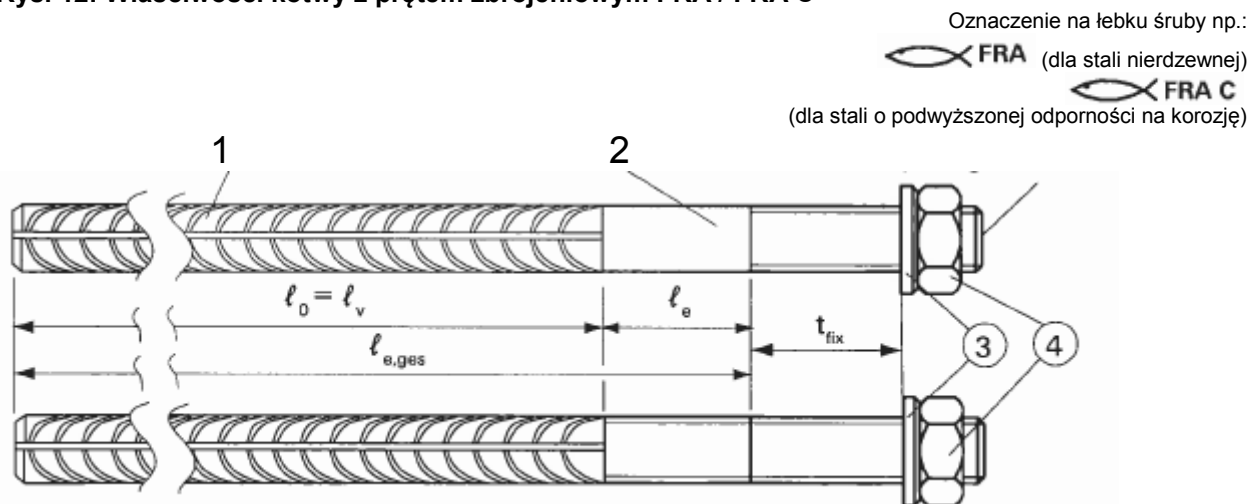
Rys. 12: Właściwości kotwy z prętem zbrojeniowym FRA / FRA C
